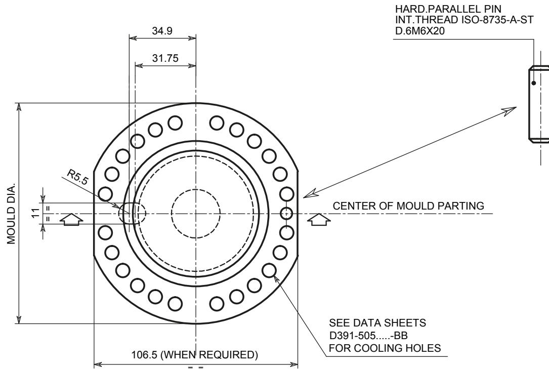
INTERLOCK TYPE Y
